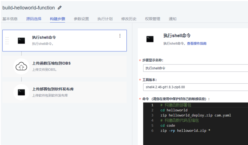
图 10-20 执行 shell 命令
