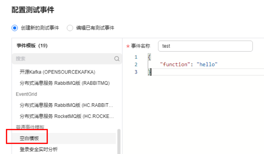
图 3-4 配置测试事件
