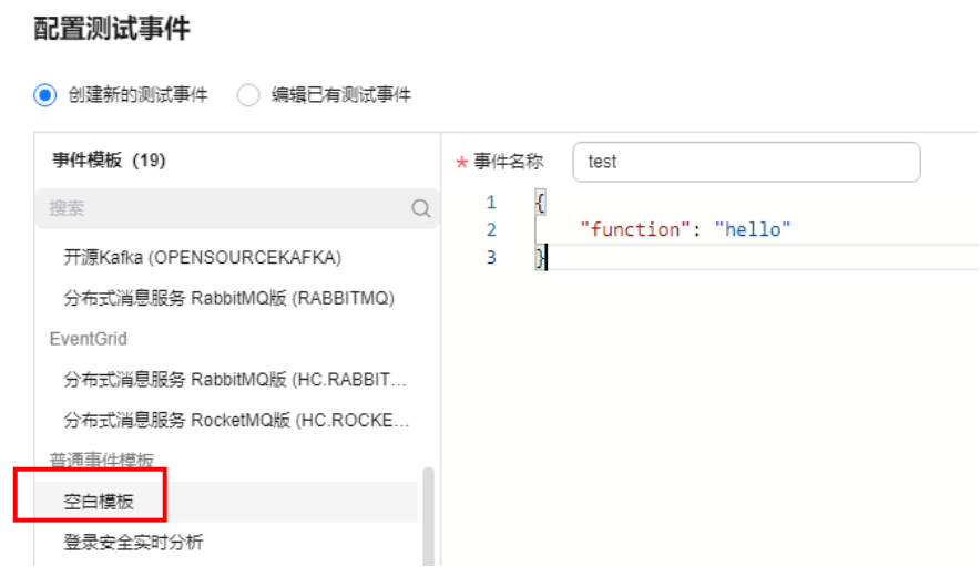
图 4-4 配置测试事件
