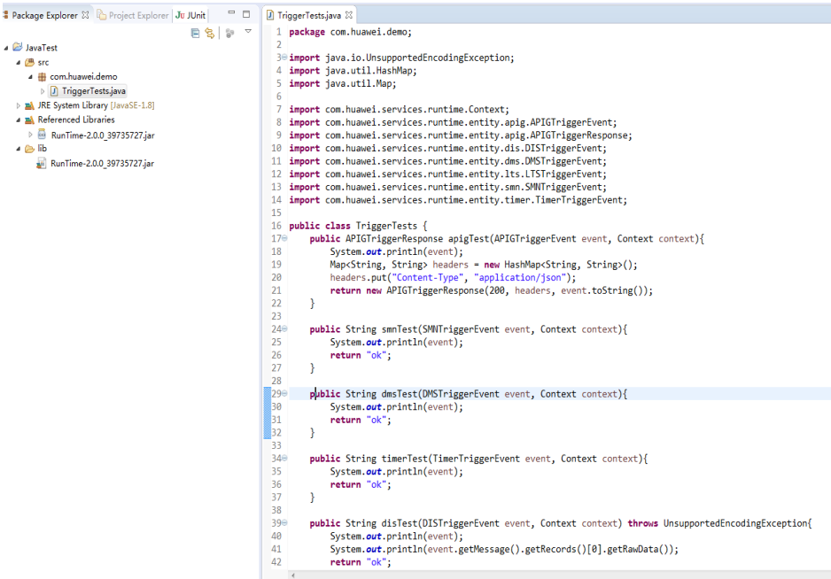
图 5-5 定义函数运行入口
